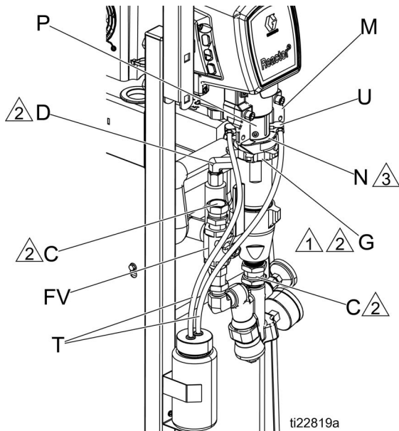
그림 1: 펌프 A
