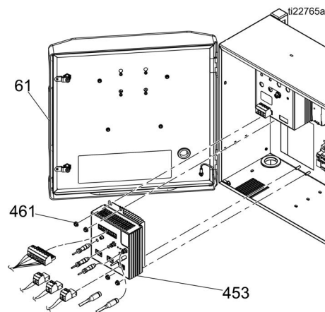
그림 21: TCM 교체
