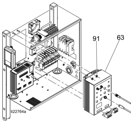
그림 20: MCM 교체
