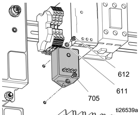
그림 19: 서지 보호장치
