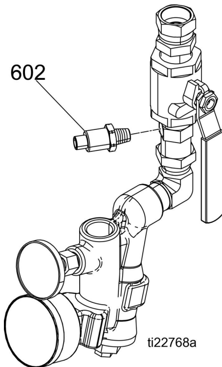
그림 6: 유체 흡입구 센서
